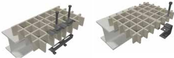
Doppelklemme Roststoßverbinder
