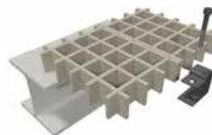
Roststoßverbinder
