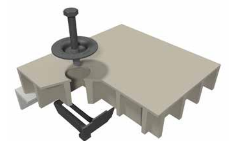
Klemme T M0436
