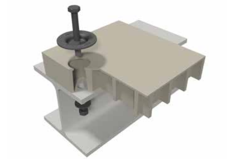
Direktverschraubung M0400
