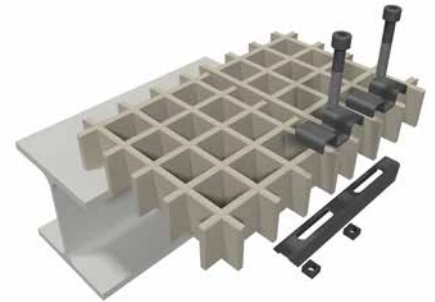
Doppelklemme V M7440
