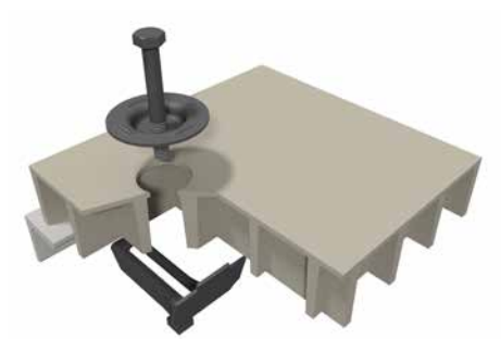
Klemme T M0442
