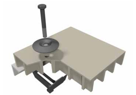
Klemme T M2936
