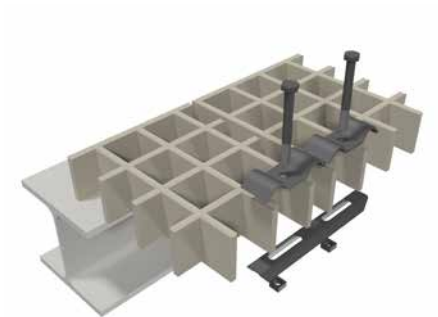
Doppelklemme V M1440
