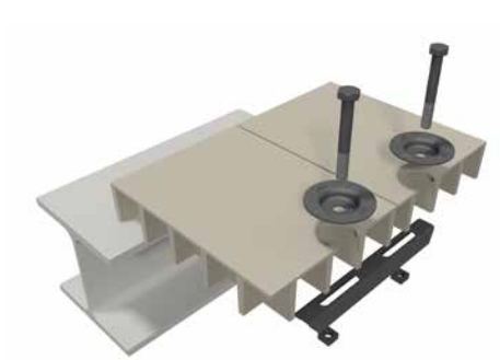
Doppelklemme V M0440
