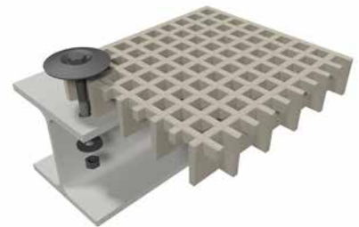
Direktverschraubung T M2900
