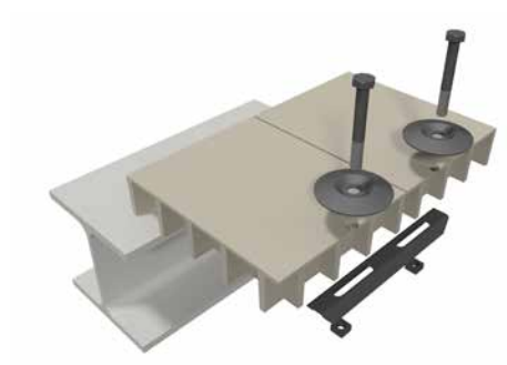
Doppelklemme V M2940
