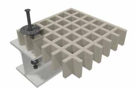
Direktverschraubung T M8600
